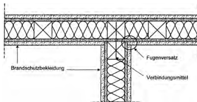
Abb. 3: Anschluss Wand an Wand mit Fugenversatz (Quelle: Prinzipskizze 4a aus MHolzBauRL bzw. Bild 5 aus M-HFHolzR)
